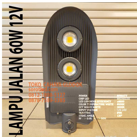
Lampu Jalan 60W 12V 24V BRIDGELUX Lumen +6600
